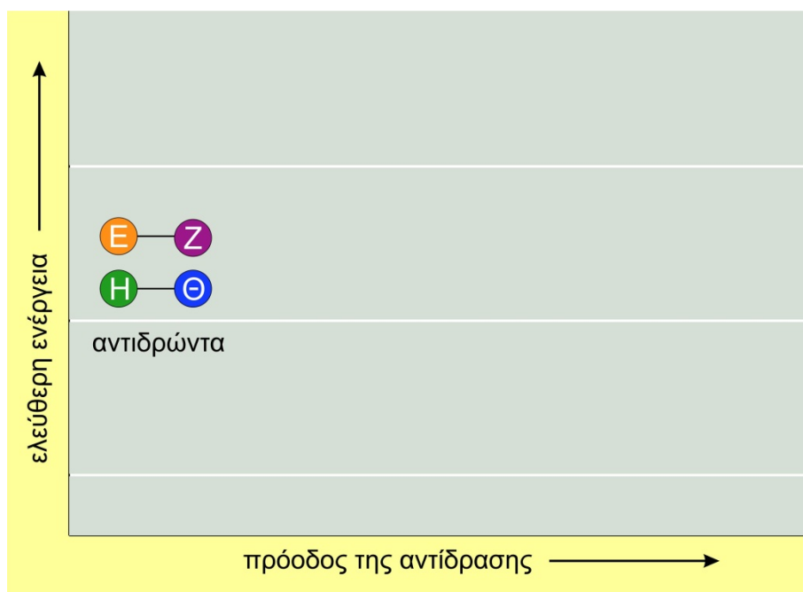
Εικόνα 2: Ενδόθερμη αντίδραση
