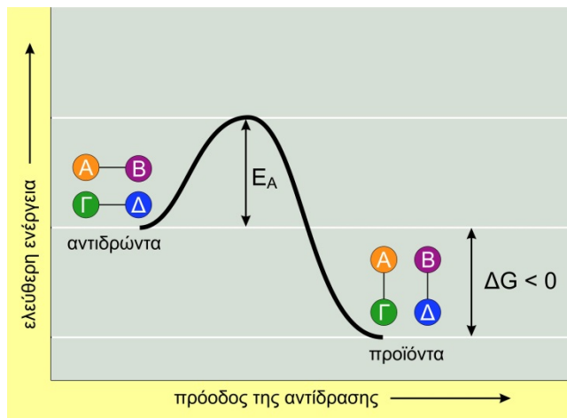
Εικόνα 1: Εξώθερμη αντίδραση
